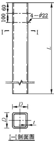
图 8 方管立柱
