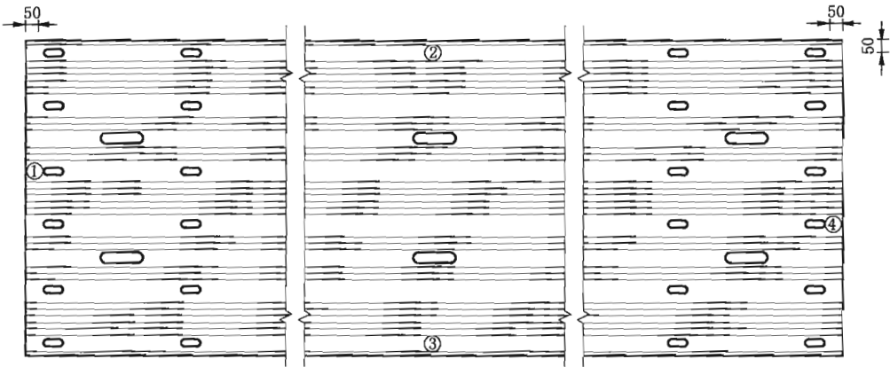
图 19 测量点位置
