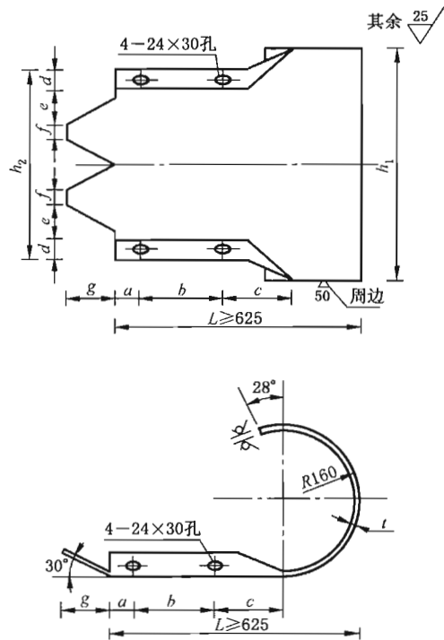
图 14 A 型端头
