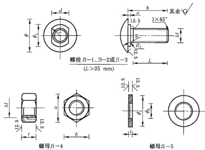
图 16 拼接螺栓
