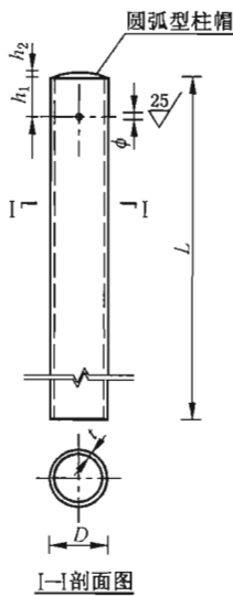
图 7 钢管立柱
