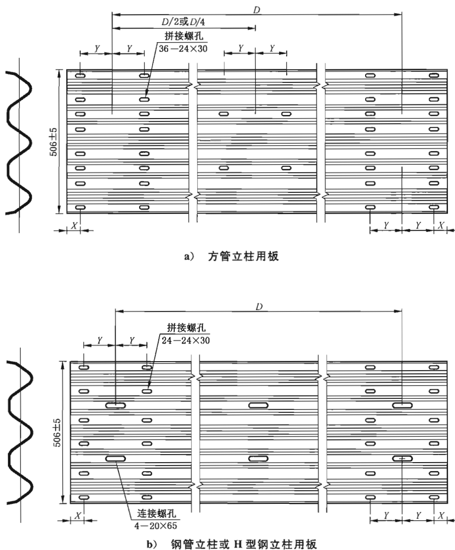
图 1 三波形梁板
